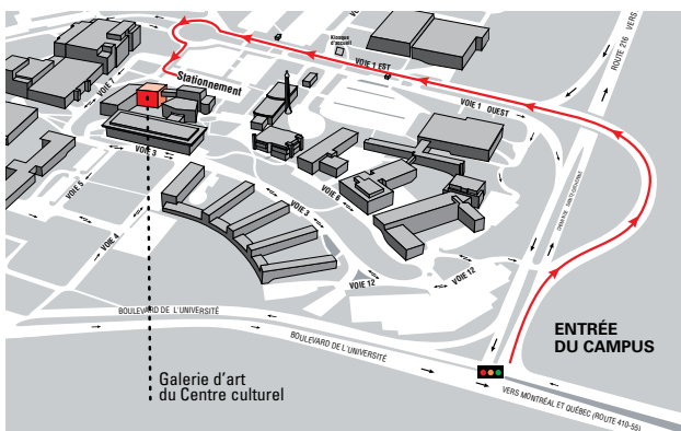
Plan partiel du Campus ouest
